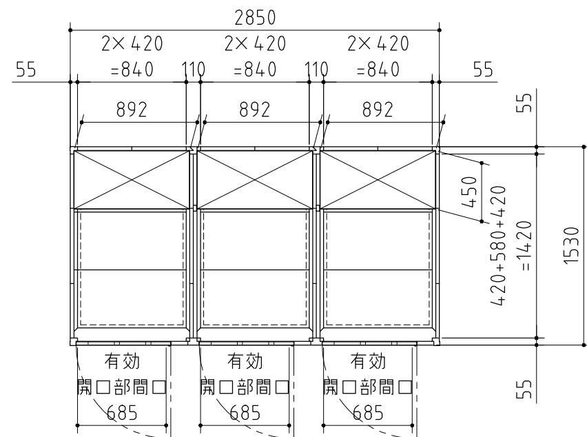
平面図
