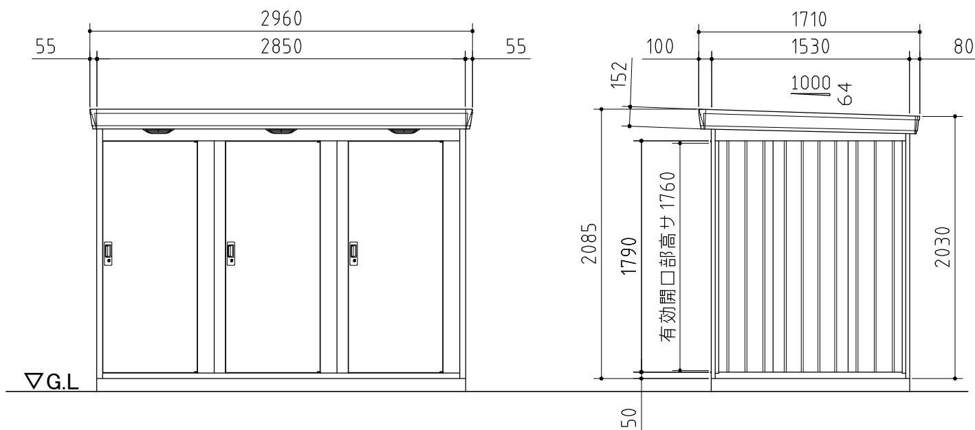
正面図
